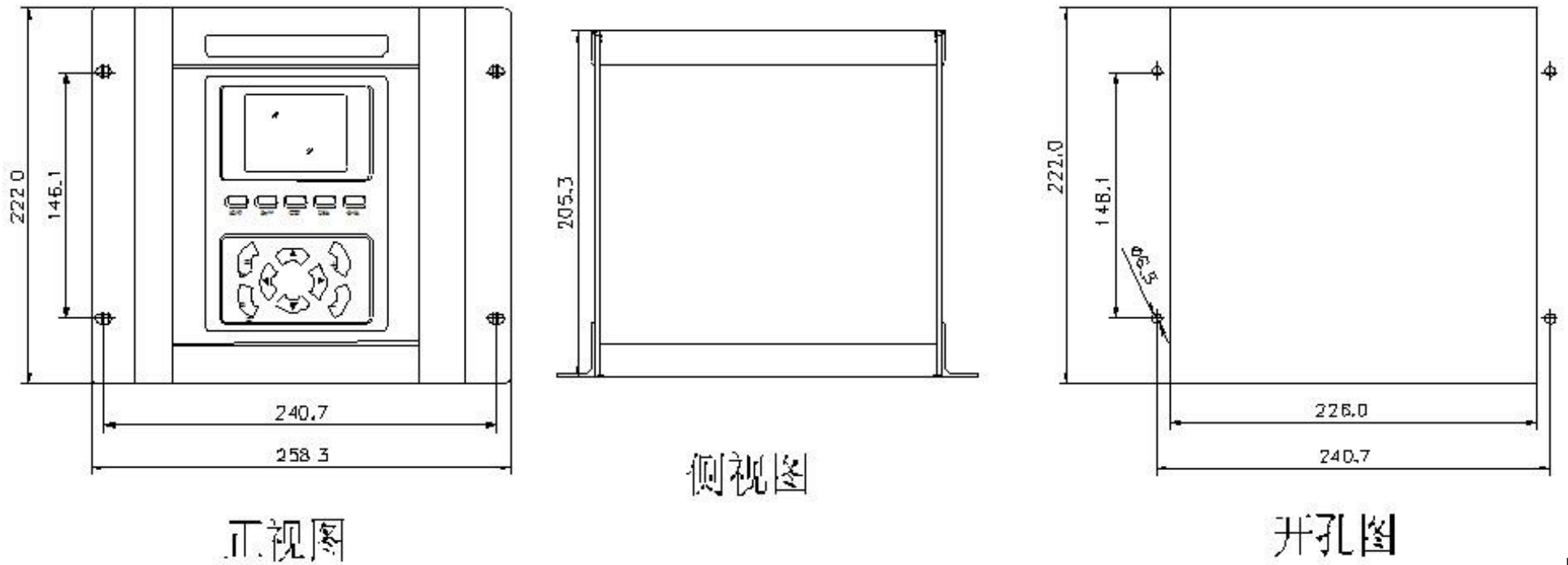
1.1 DPY-3 系列频率电压紧急控制装置外型尺寸及开孔图
